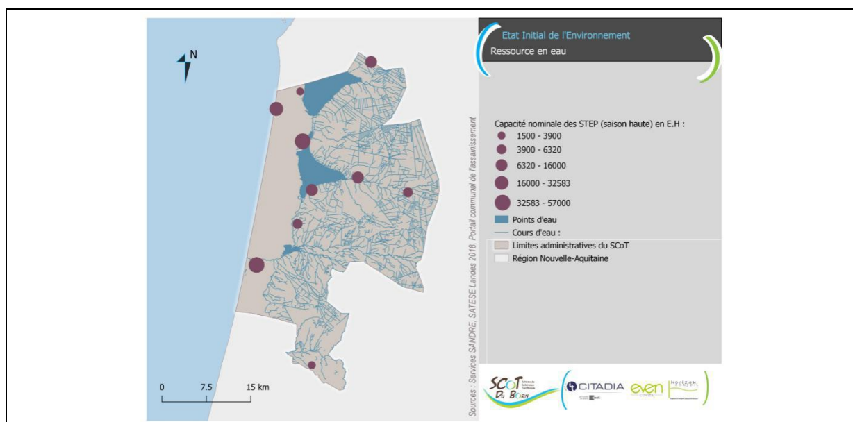
FIGURE 50 : CARTE DES STRUCTURES D'ASSAINISSEMENT
